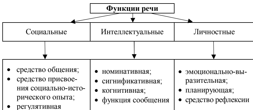
Рис.1. Классификация функций речи (И.А.Зимняя)
