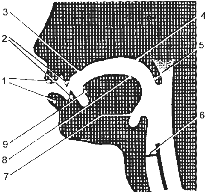
Рис. 18. Профиль органов артикуляции: 1 — губы, 2 — резцы, 3 — альвеолы, 4 — твердое нёбо, 5 — мягкое нёбо, 6 — голосовые складки, 7 — корень языка, 8 — спинка языка, 9 — кончик языка
